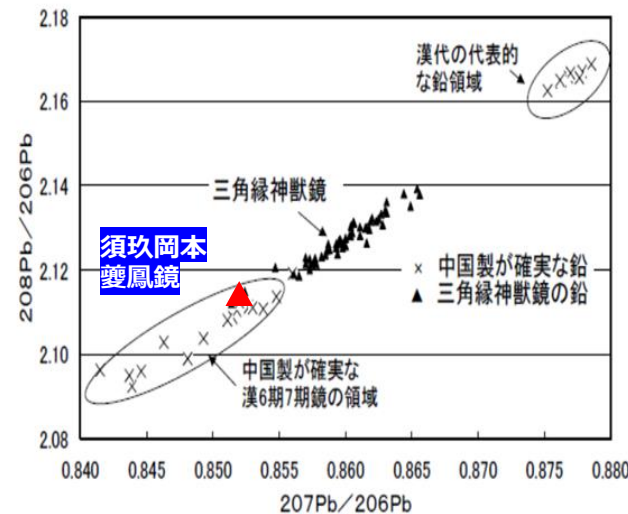
図6 中国製が確実な鉛原料と三角縁神獸鏡の関係(A式)
